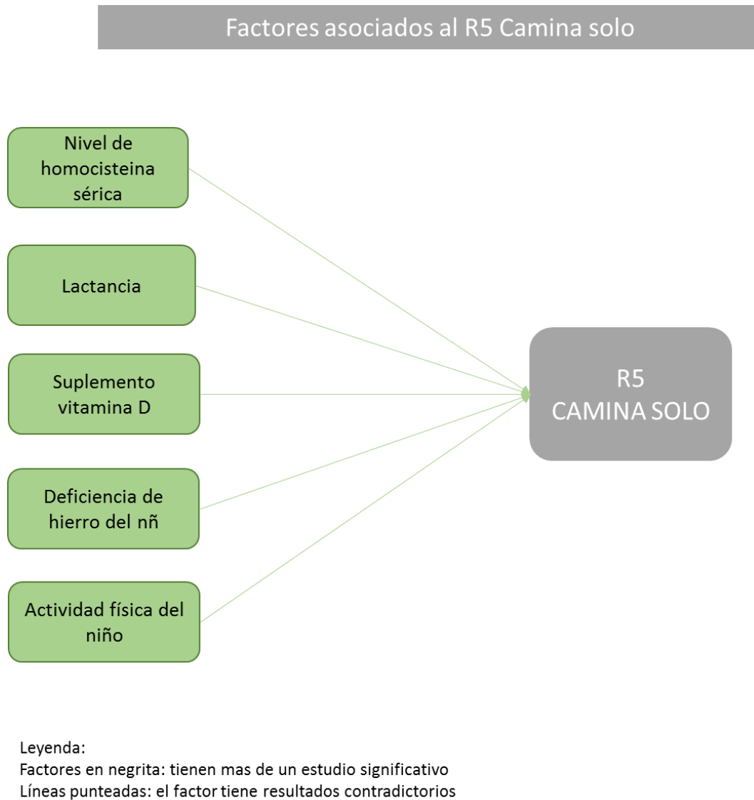
Gráfico 5. Redes nomológicas para el R5 Camino solo
