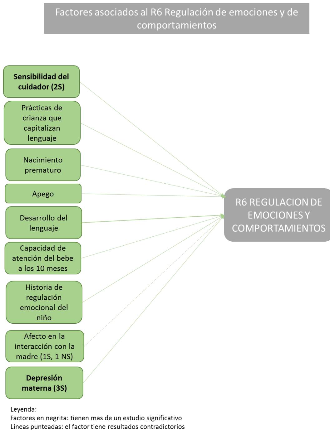
Gráfico 6. Redes nomológicas para el R6 Regulación de emociones y comportamientos
