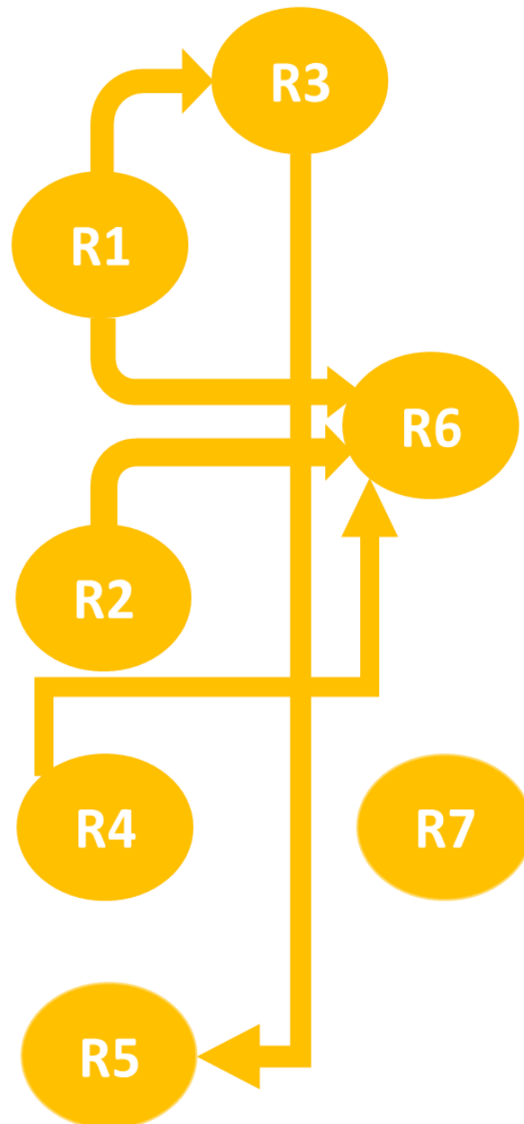
Gráfico 8. Relaciones entre resultados del DIT, según la revisión sistemática
