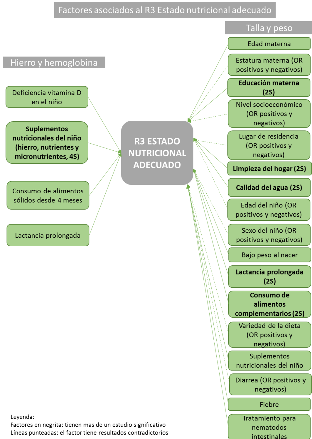
Gráfico 3. Redes nomológicas para el R3 Estado nutricional adecuado
