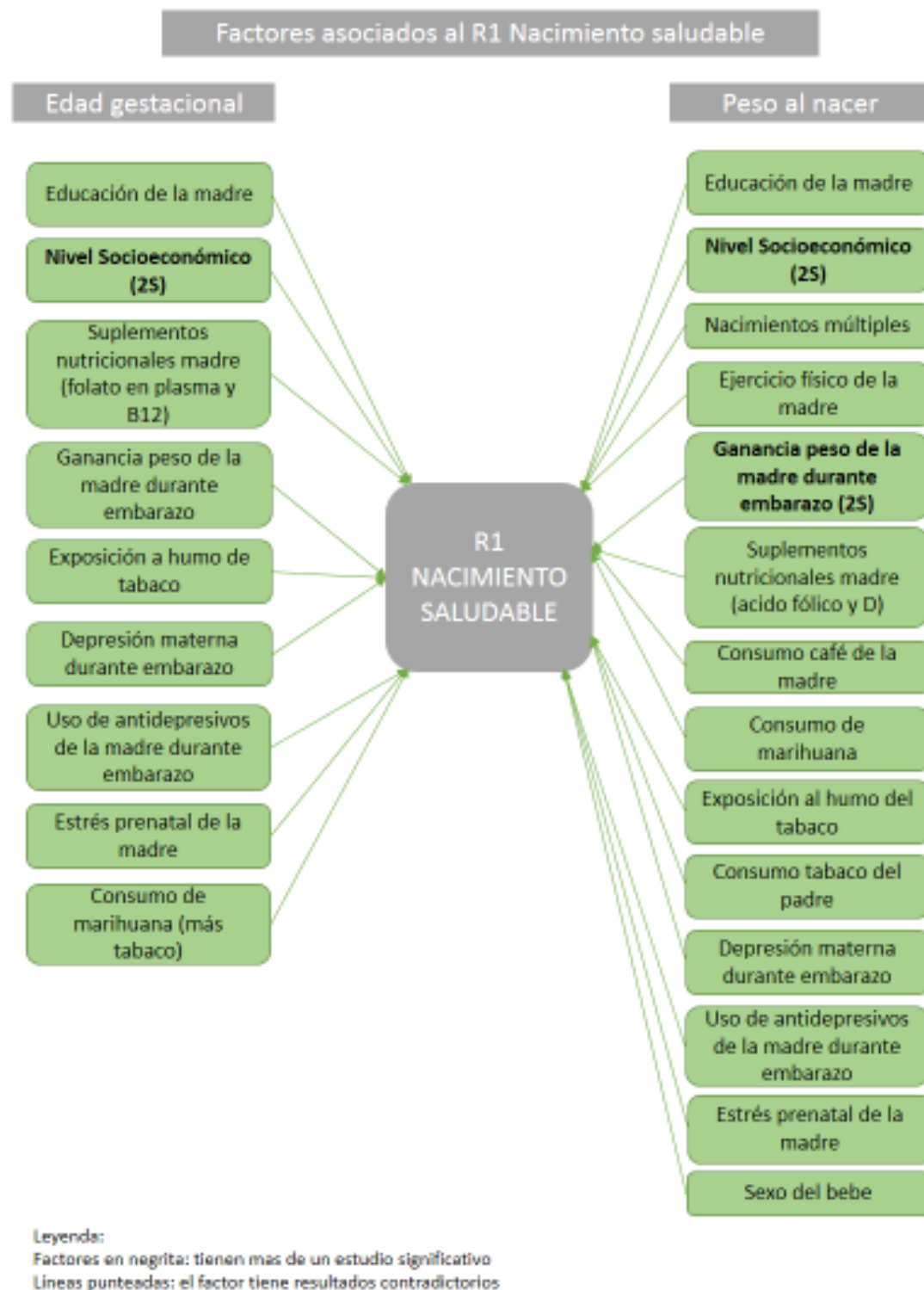
Gráfico 1. Redes nomológicas para el R1 Nacimiento saludable
